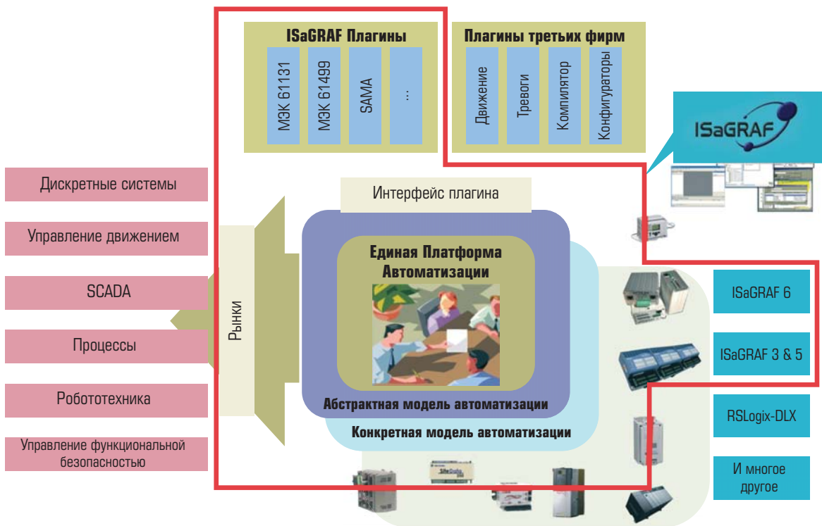
Рис. 1. Общий взгляд на Единую Платформу Автоматизации
