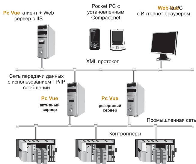
Рис. 2. Пример архитектуры PcVue: система с Web-клиентами
