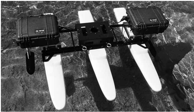
Рис. 5. Робот на воде Kingfisher M100 с бортовым компьютером fit-PC2
