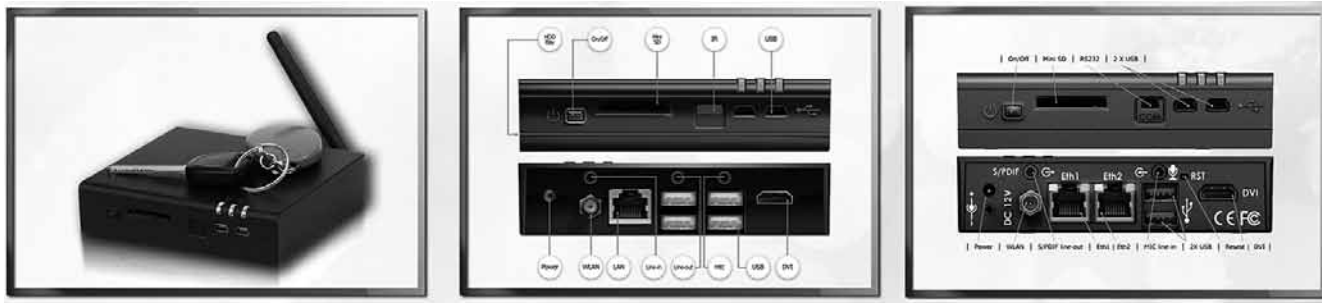
Рис. 1. Внешний вид fit-PC2 и fit-PC2i
