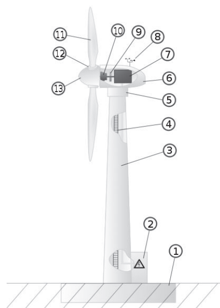
Рис. 1. Схема ветрогенератора
