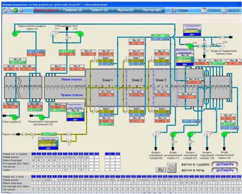
Рис. 3. Экран «инемосхема»
